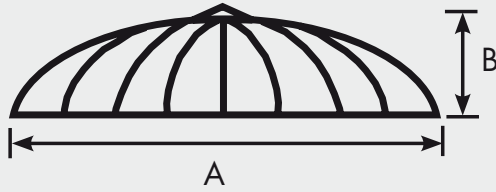
Zeppeliinipääty
