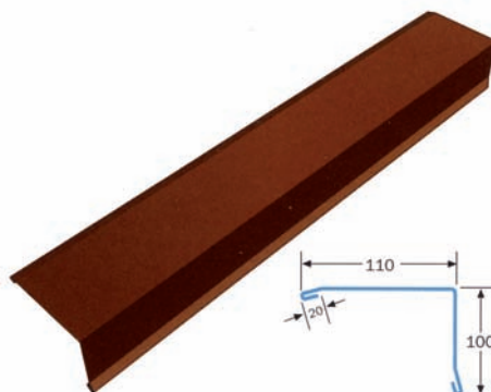
Päätylista
