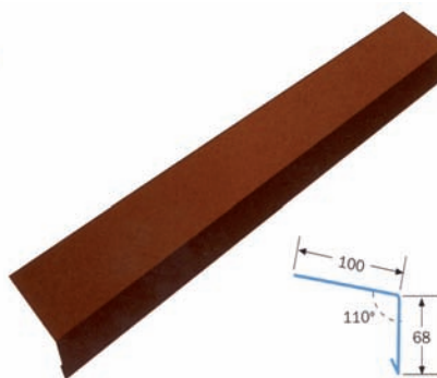
Räystäalista
