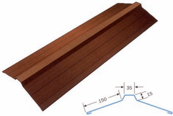
Harjalista, sileä
