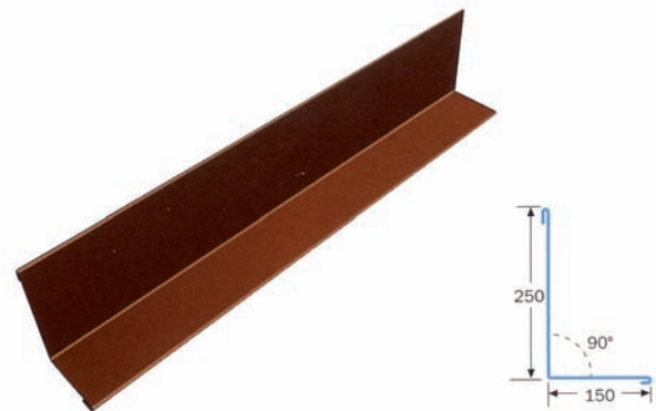
Liitoslista
