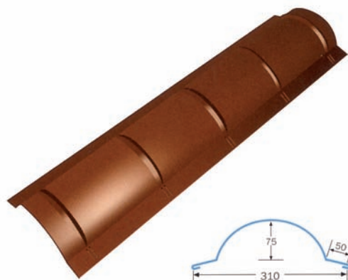
Harjalista, pyöreä
