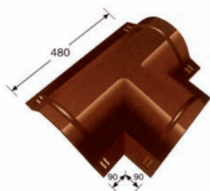
T-haara
