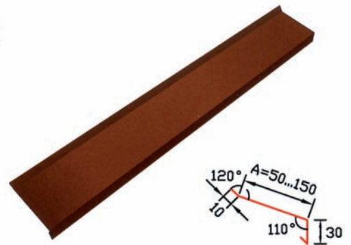
Ikkunan alalista
