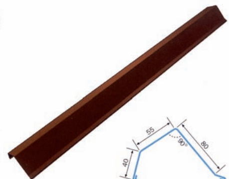
Päätylista Modern
